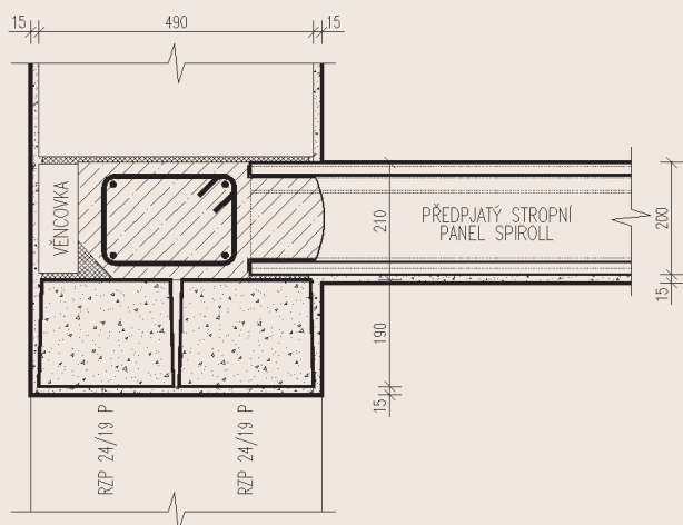
nezateplené nadpraží var. 2
