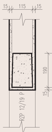
TLOUŠŤKA ZDIVA 115 mm
