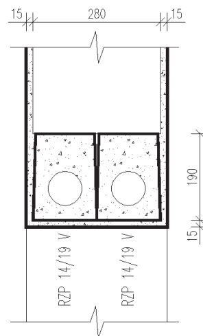
TLOUŠŤKA ZDIVA 280 mm
