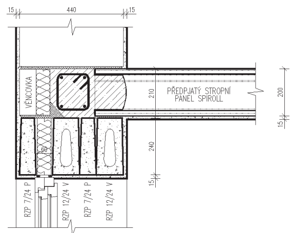
zateplené nadpraží var. 1
