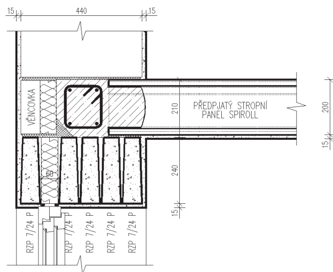
zateplené nadpraží var. 2
