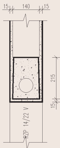
TLOUŠŤKA ZDIVA 140 mm
