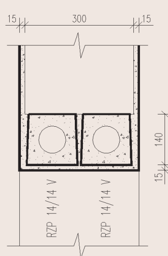
TLOUŠŤKA ZDIVA 300 mm
