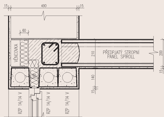
TLOUŠŤKA ZDIVA 490 mm
