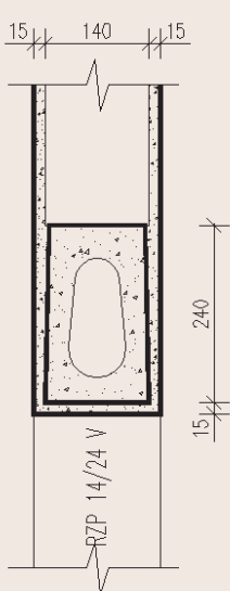
TLOUŠŤKA ZDIVA 140 mm
