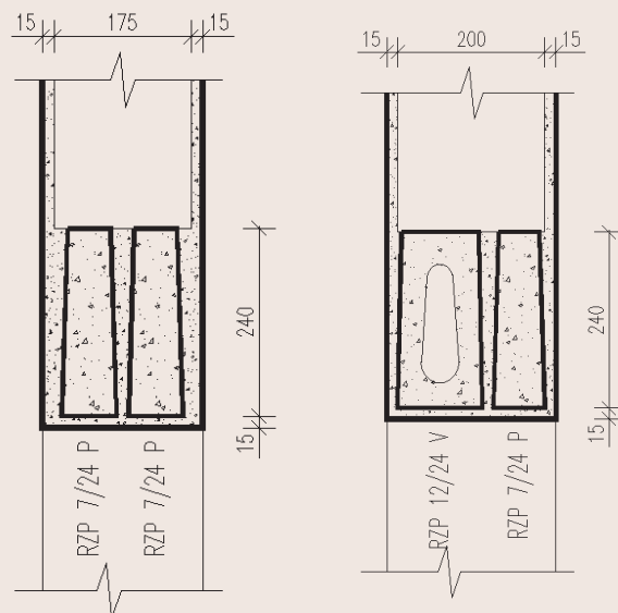
TLOUŠŤKA ZDIVA 200 mm
