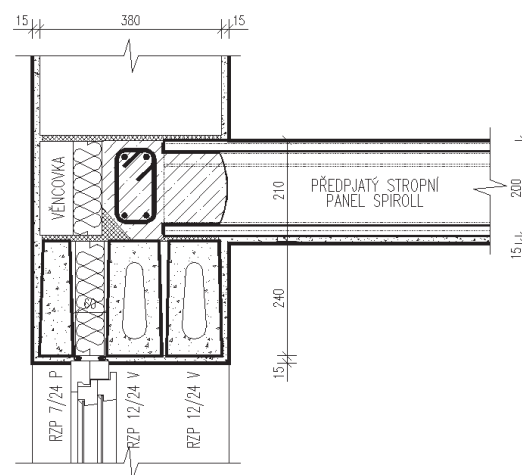
zateplené nadpraží
