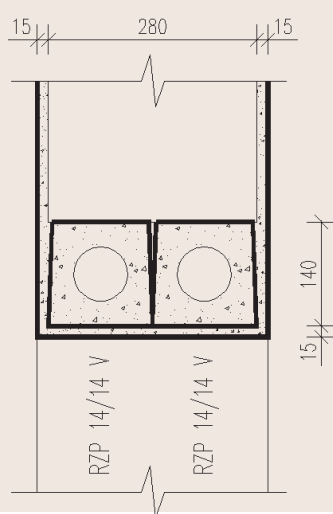
TLOUŠŤKA ZDIVA 280 mm
