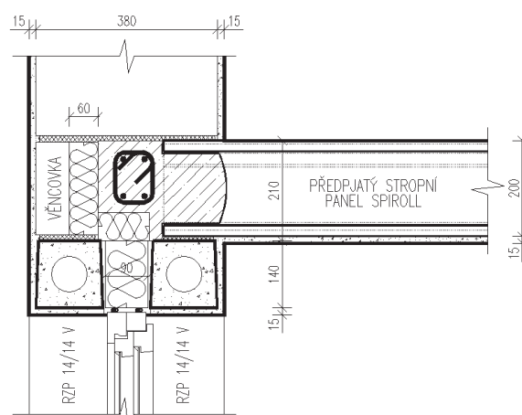
TLOUŠŤKA ZDIVA 380 mm
