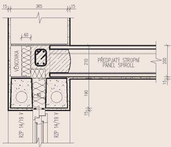
zateplené nadpraží
