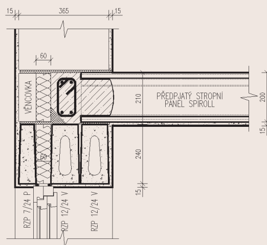
zateplené nadpraží
