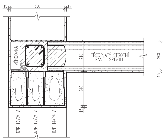
nezateplené nadpraží
