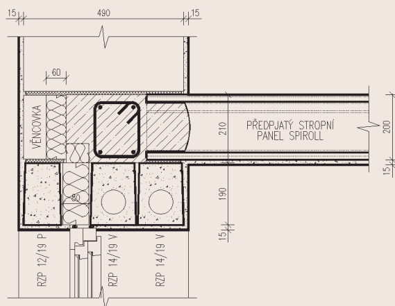
zateplené nadpraží
