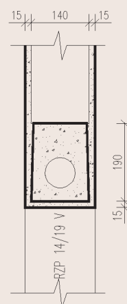
TLOUŠŤKA ZDIVA 140 mm
