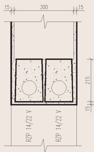
TLOUŠŤKA ZDIVA 300 mm
