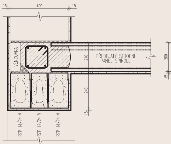
nezateplené nadpraží
