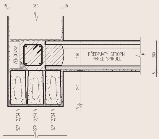
nezateplené nadpraží
