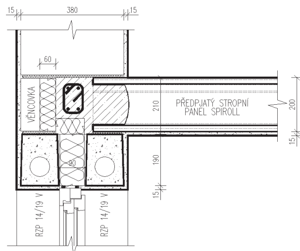
zateplené nadpraží
