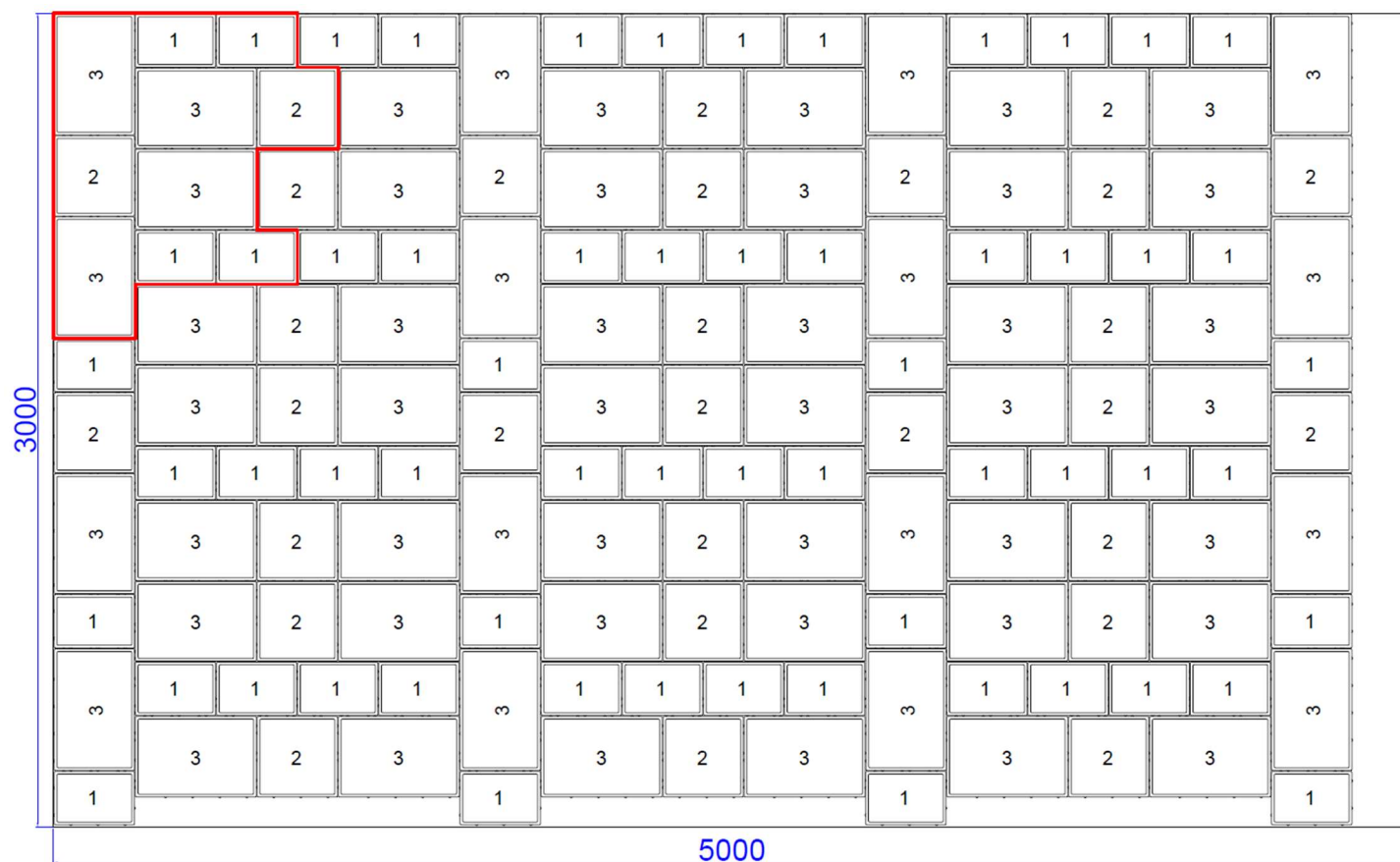
Obr. 3 – Návrh skladby položení dlažby Moravský granit se souvislými spárami
